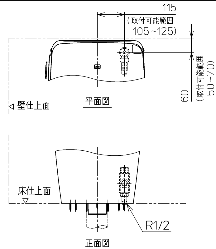
床給水仕様の場合
